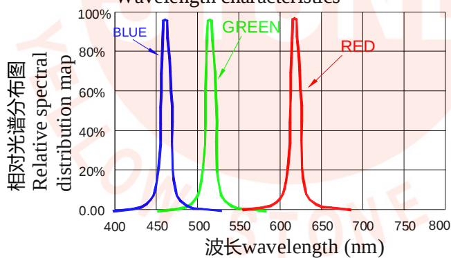
波长特性
