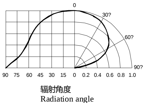
典型的辐射方向图 120°
