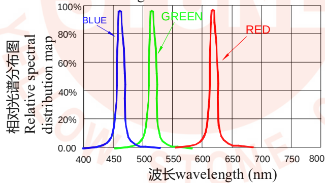
波长特性
