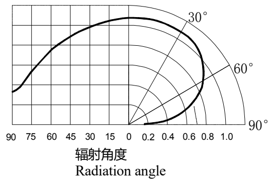
典型的辐射方向图 160°
