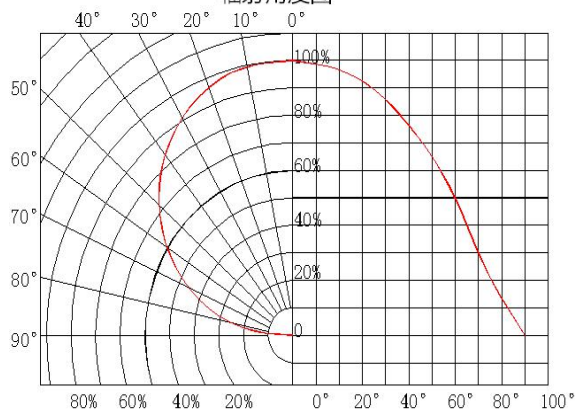
Radiation diagram 辐射角度图
