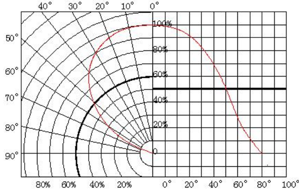
Radiation diagram 辐射角度图
