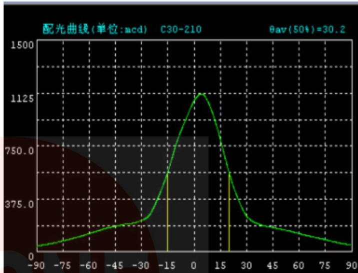
Light intensity distribution curve 光强分布曲线[直角坐标] (单位: mcd)
