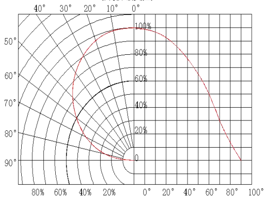
Radiation diagram 辐射角度图
