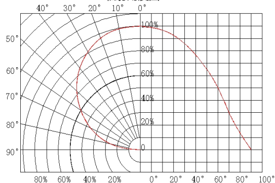
辐射角度图
