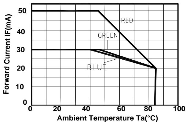
8). Thermal Design
