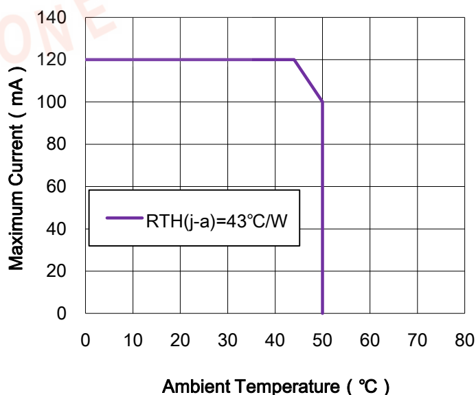
(4) 电流与环境温度 CURRENT VS. AMBIENT TEMPERATURE
