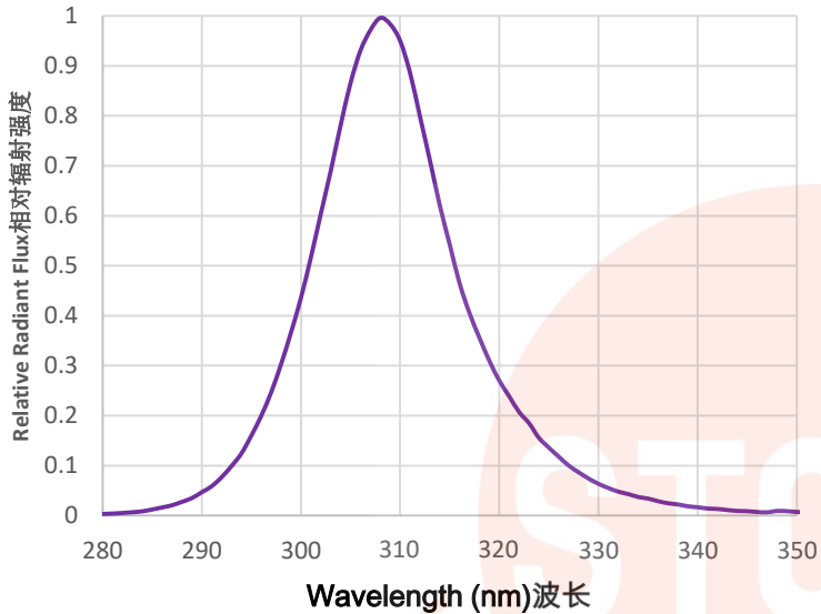
(1) 相对光谱分布 Relative spectral distribution
