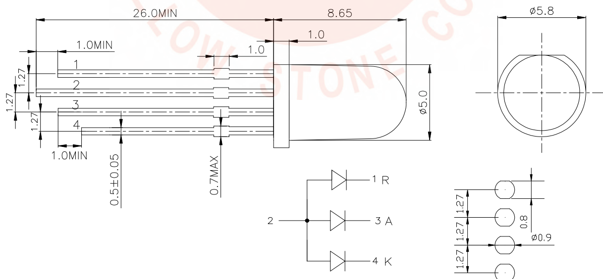
焊盘推荐图
